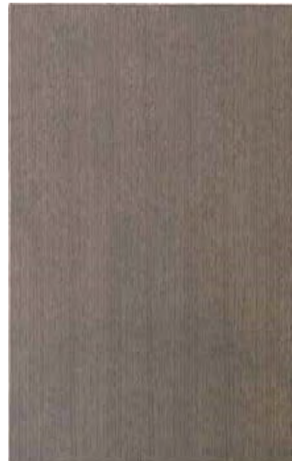
Astoria
